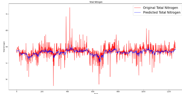
Figure 10d. Actual Vs Predicted Total Nitrogen.
